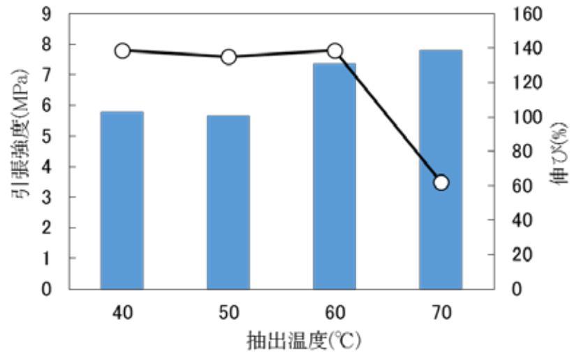
図 抽出温度とケラチンフィルムの引張強度、伸びの関係 (ケラチン/グリセリン = 5/1) : 引張強度 ■ : 伸び
