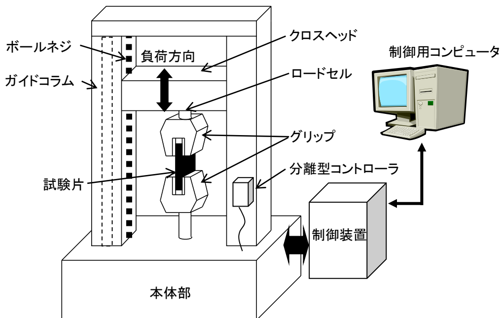
図 材料試験機の構成
