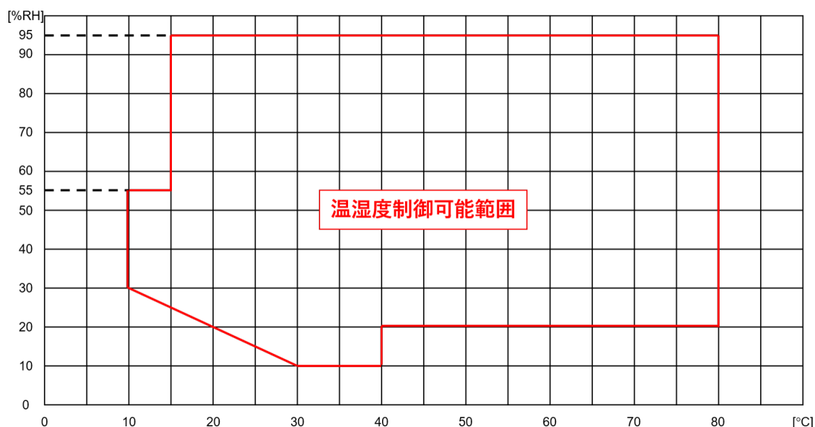
図 温湿度制御可能範囲図
